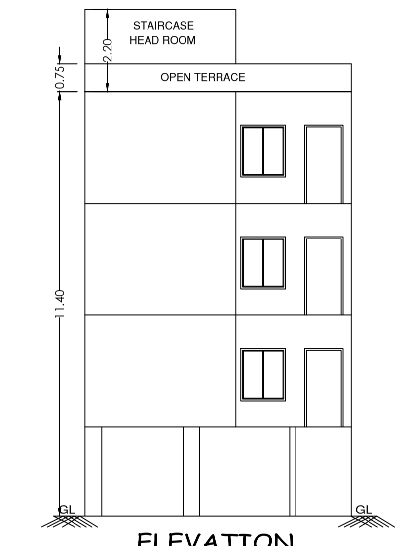
ELEVATION
